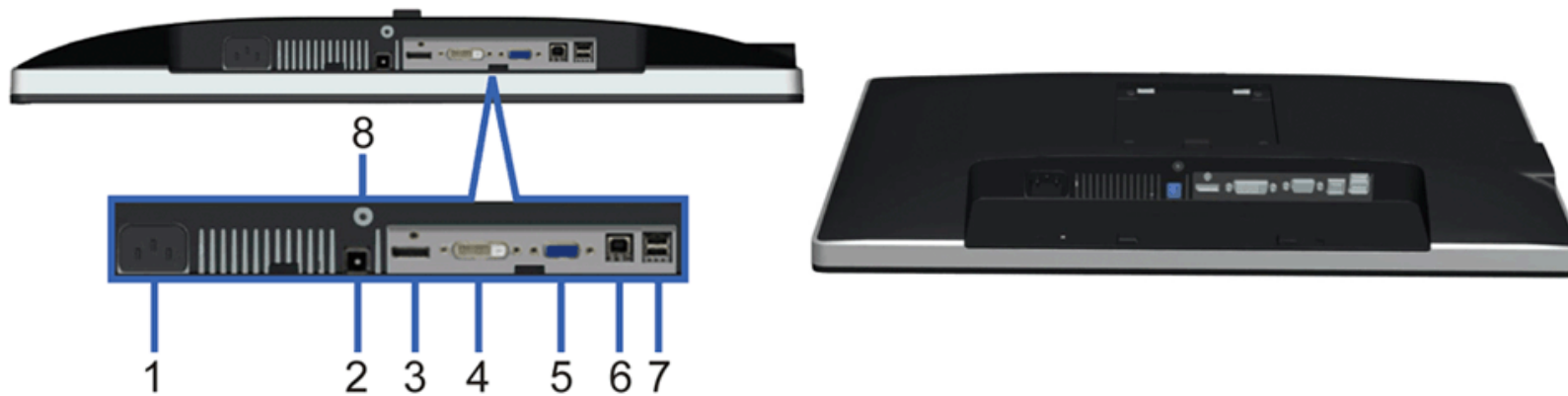
Vista inferior
